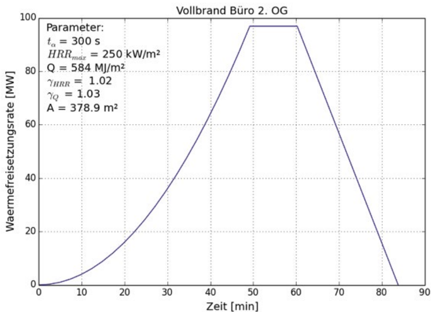
Abbildung 8: Wärmefreisetzungsrates für das Szenario „Standsicherheit im Brandfall“
